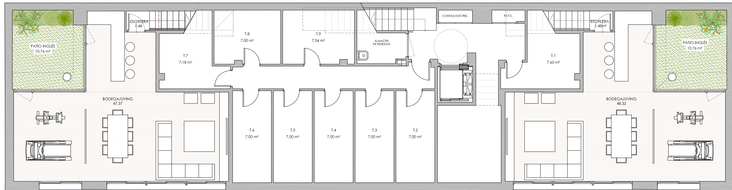
PLANTA SEMISÓTANO
